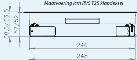
Maatvoering icm RVS T25 klapdeksel
